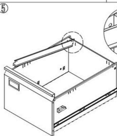
Paigaldage riputusvardad.
