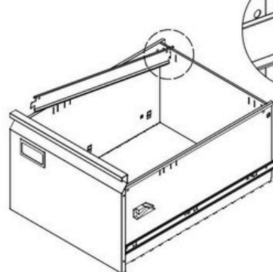
Nainštalujte závesné tyče.
