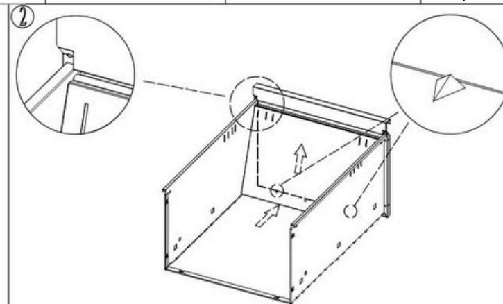
Paigaldage sahtli eesmine tihend vastavalt joonisele.
