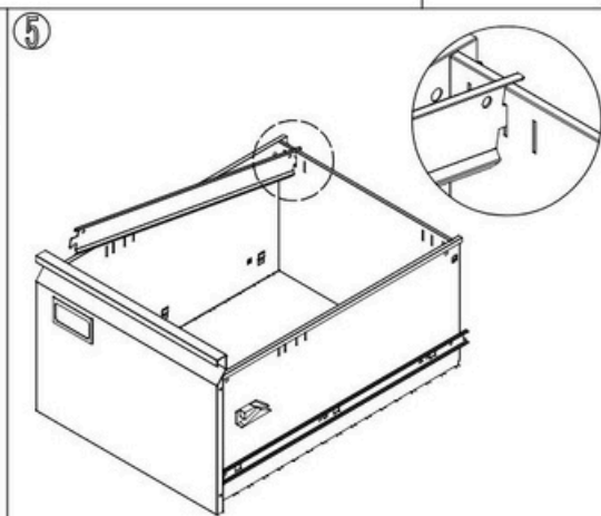
Montare le aste di sospensione.
