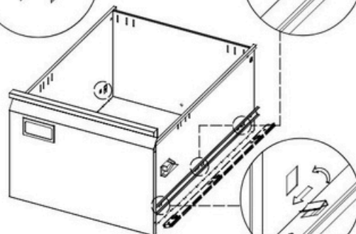
Montez les glissières intérieures.
