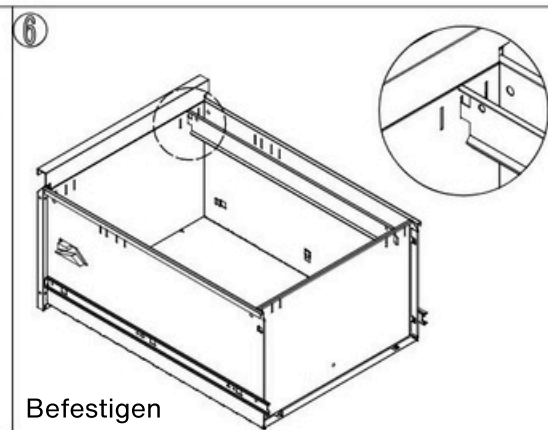
Montieren Sie die vordere Schubladendichtung gemäß der Abbildung.
