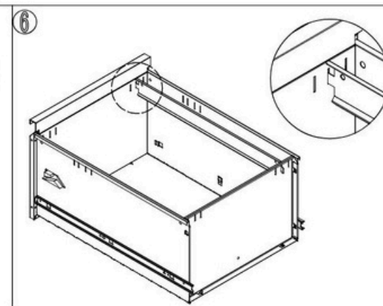
Fäst upphängningsstängerna på lådpanelerna enligt bilden.
