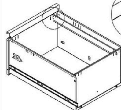
Rögzítse a függesztőrudakat a fiókelőlapokhoz az ábrának megfelelően.
