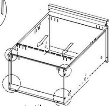
Asenna laatikon etupaneeli kuvan mukaisesti.
