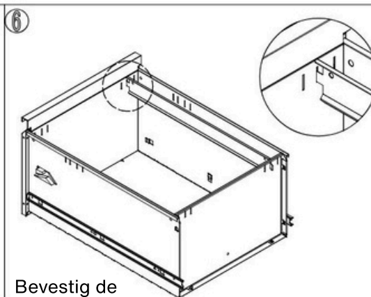
Monteer de voorste ladeafdichting zoals weergegeven op de afbeelding.
