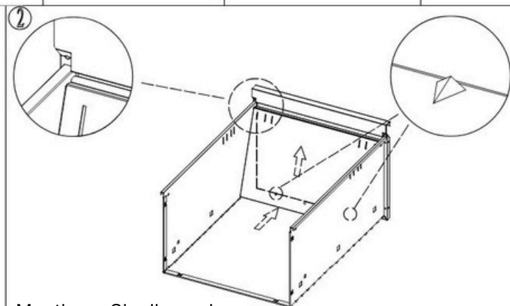
Montieren Sie die vordere Schubladendichtung gemäß der Abbildung.
