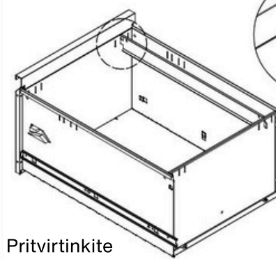
Sumontuokite priekinį stalčiaus sandariklį, kaip parodyta paveikslėlyje.
