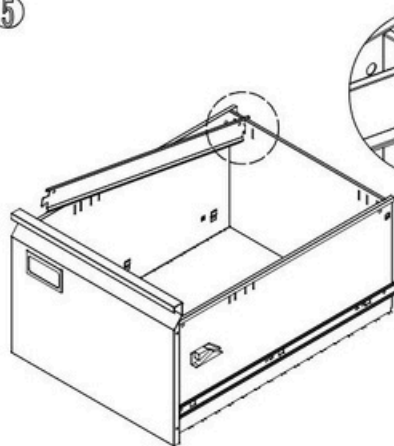
Montez les barres de suspension.
