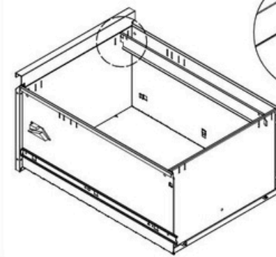
Upevnite závesné tyče k panelom zásuviek, ako je znázornené na obrázku.
