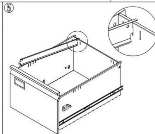
Монтирайте лостовете за окачване.
