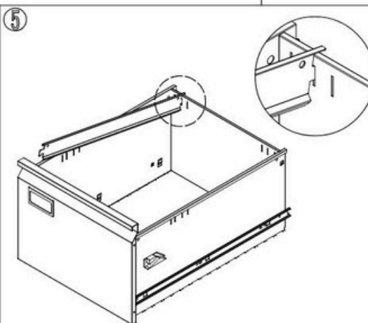
Montați barele de suspendare.
