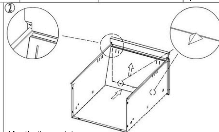
Montirajte prednju brtvu ladice kao što je prikazano na slici.
