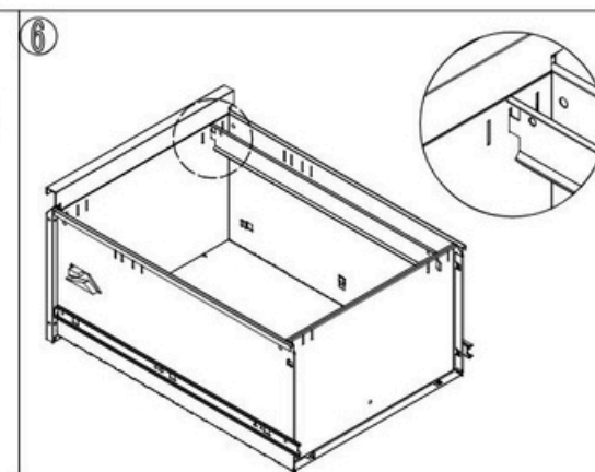
Obešalne palice pritrdite na panele predalov, kot je prikazano na sliki.
