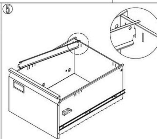
Namestite obešalne palice.
