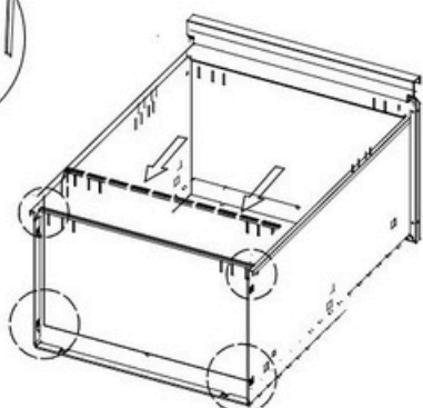
Montez la façade du tiroir comme indiqué sur l'image.
