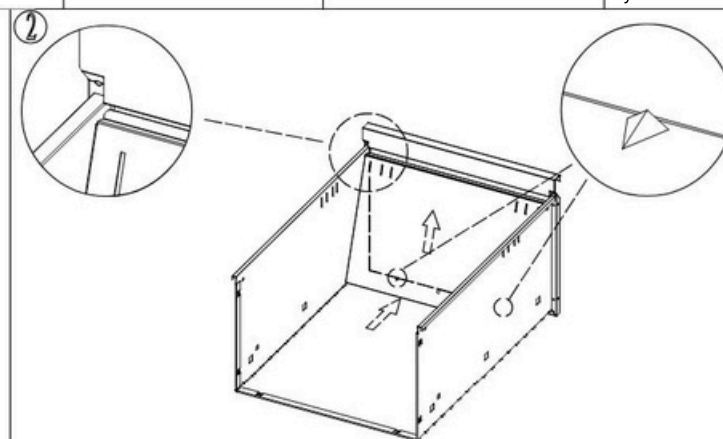
Montera den främre lådtätningen enligt bilden.
