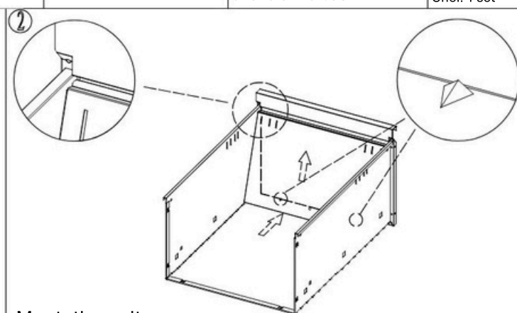
Montați garnitura frontală a sertarului conform imaginii.
