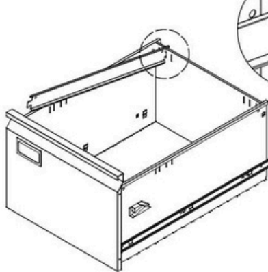
Monte as barras de suspensão.
