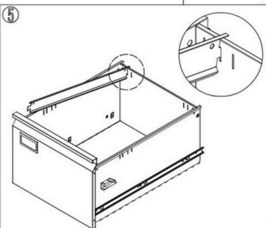
Montirajte šipke za vješanje.
