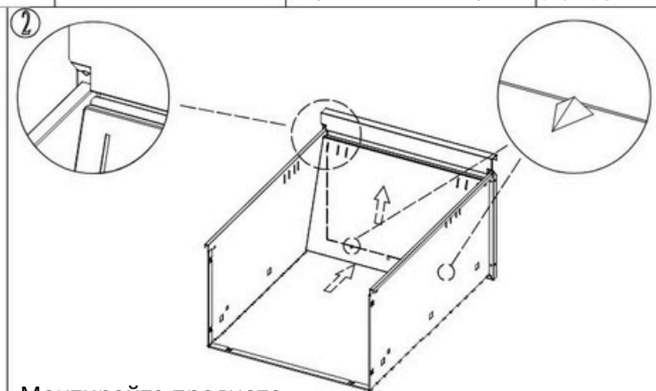
Монтирайте предното уплътнение на чекмеджето според изображението.
