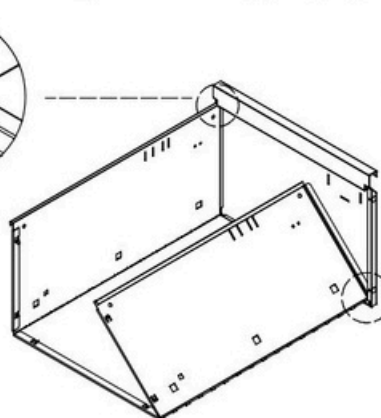
Установите складной короб ящика.
