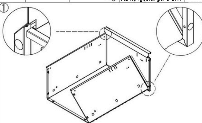
Montieren Sie die klappbare Schubladenbox.
