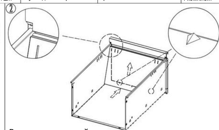
Встановіть передній ущільнювач шухляди, як показано на зображенні.
