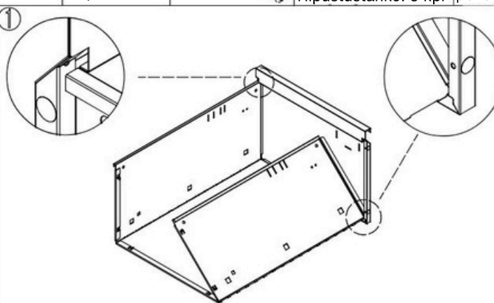
Lukitustanko: 1 kpl
