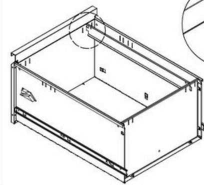
Kiinnitä ripustustangot laatikon paneeliin kuvan mukaisesti.
