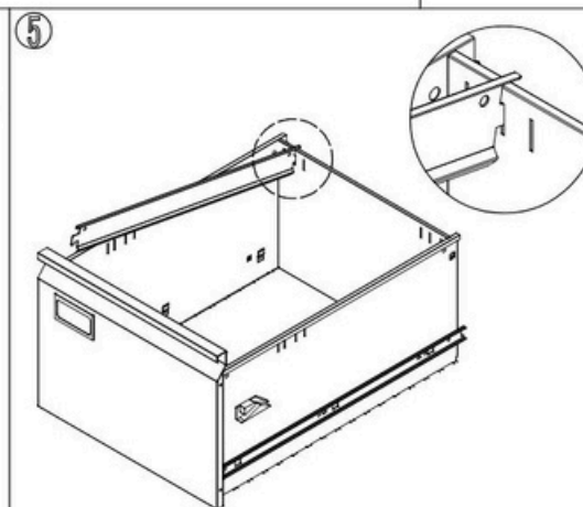
Montera upphängningsstängerna.
