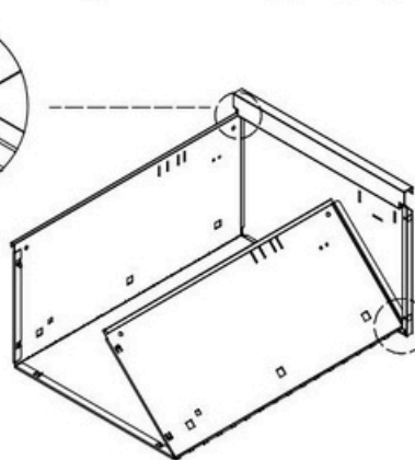
Monter den sammenfoldelige skuffeboks.
