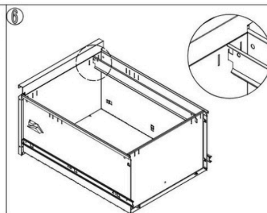
Pričvrstite šipke za vješanje na ploče ladica kao što je prikazano na slici.
