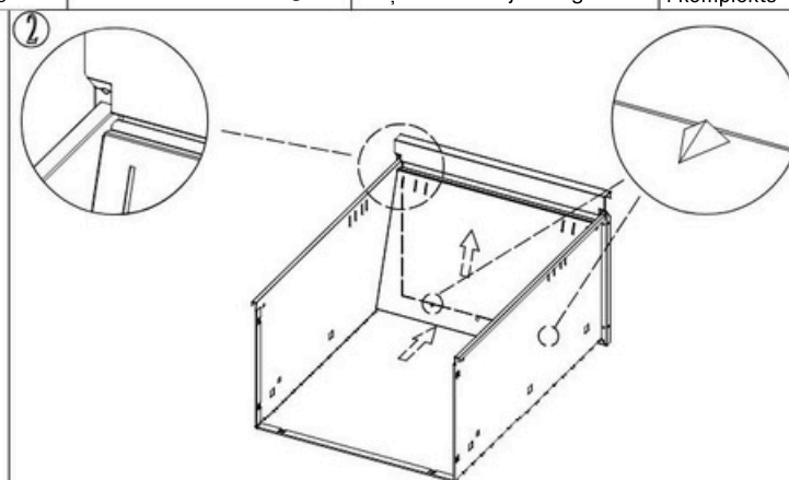
Uzstādi priekšējo atvilktnes blīvi, kā parādīts attēlā.
