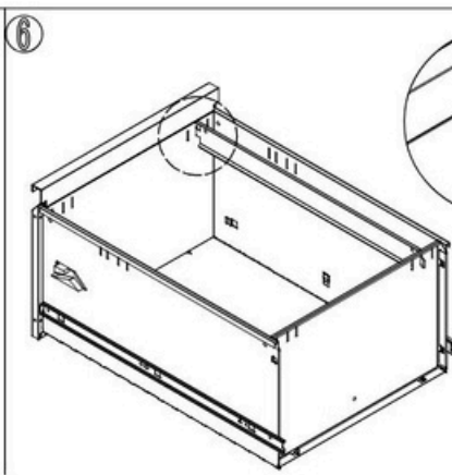
Kinnitage riputusvardad sahtlipaneelide külge vastavalt joonisele.
