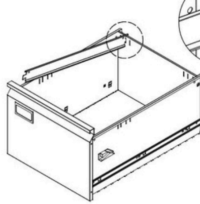
Установите штанги для подвешивания.
