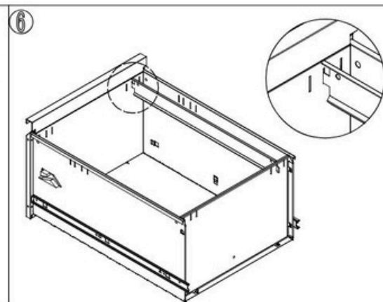
Fixați barele de suspendare pe panourile sertarelor conform imaginii.
