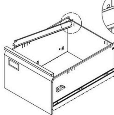
Monte las barras de suspensión.
