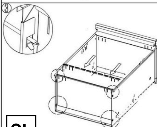
SL Namestite sprednjo ploščo predala, kot je prikazano na sliki.
