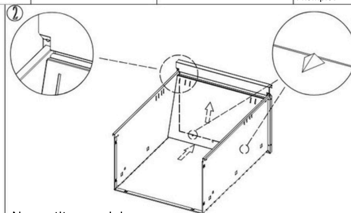
Namestite sprednje tesnilo predala, kot je prikazano na sliki.
