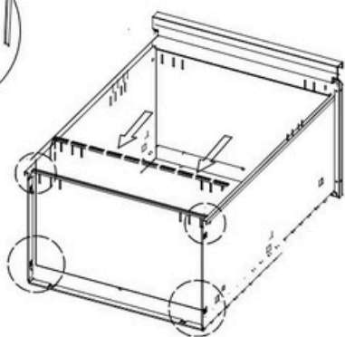
Paigaldage sahtli esipaneel vastavalt joonisele.
