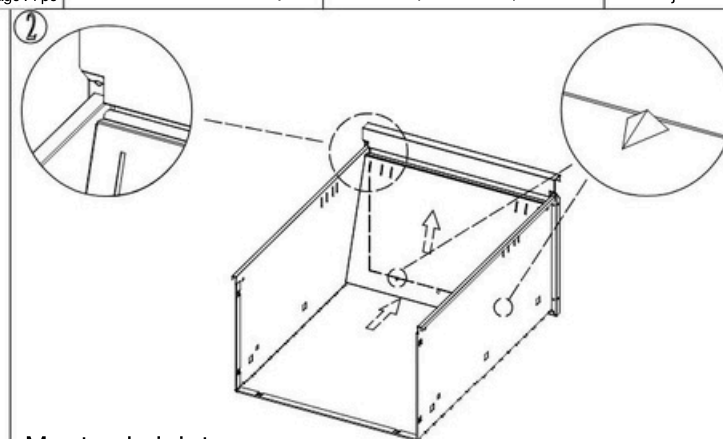
Montez le joint avant du tiroir comme indiqué sur l'image.
