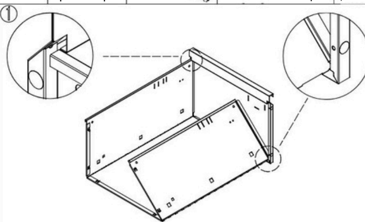
Монтирайте сгъваемия модул на чекмеджето.
