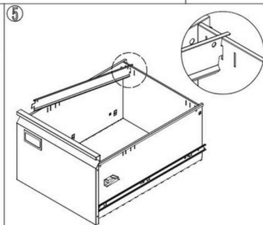
Montirajte šipke za kačenje.
