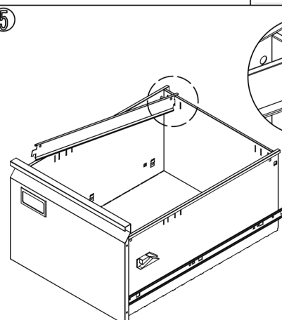
Monter opphengsstengene.
