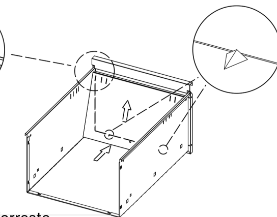
Monter det forreste skuffedæksel som vist på billedet.
