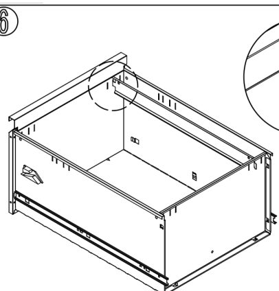
Fest opphengsstengene til skuffepanelene som vist på bildet.
