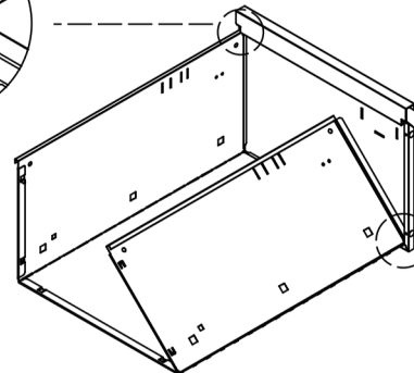
Monter den sammenleggbare skuffen.
