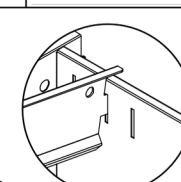
Zamontuj przednią oślonę szuflady zgodnie z rysunkiem.
