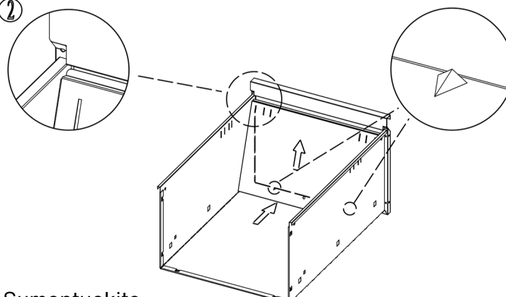
Sumontuokite priekinį stalčiaus dangtelį pagal paveikslėlį.
