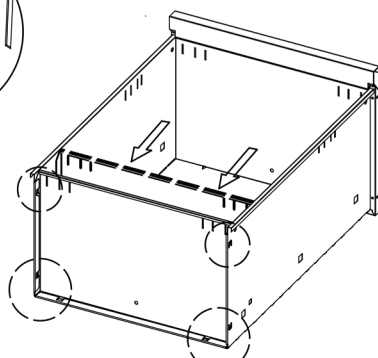
Sumontuokite stalčiaus priekinę plokštę pagal paveikslėlį.
