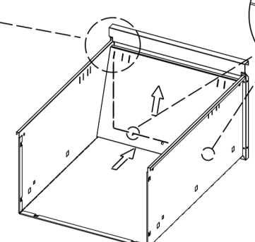
Monter det fremre skuffedekselet som vist på bildet.
