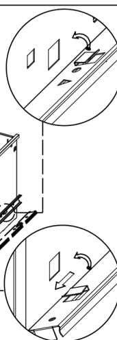
Zamontuj składaną szufladę.
